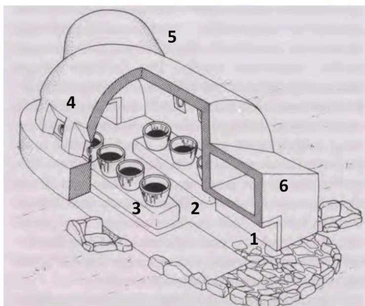
Skematisk tegning af glasovn.
